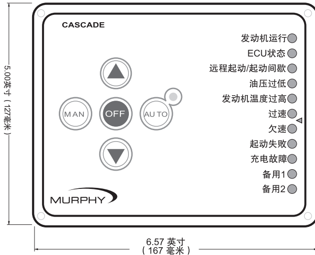
前视图
